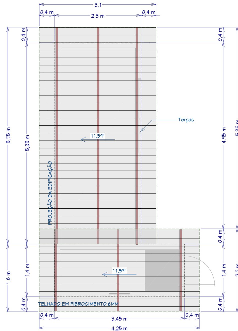
2 Planta de Cobertura 1 cm = 50 cm
