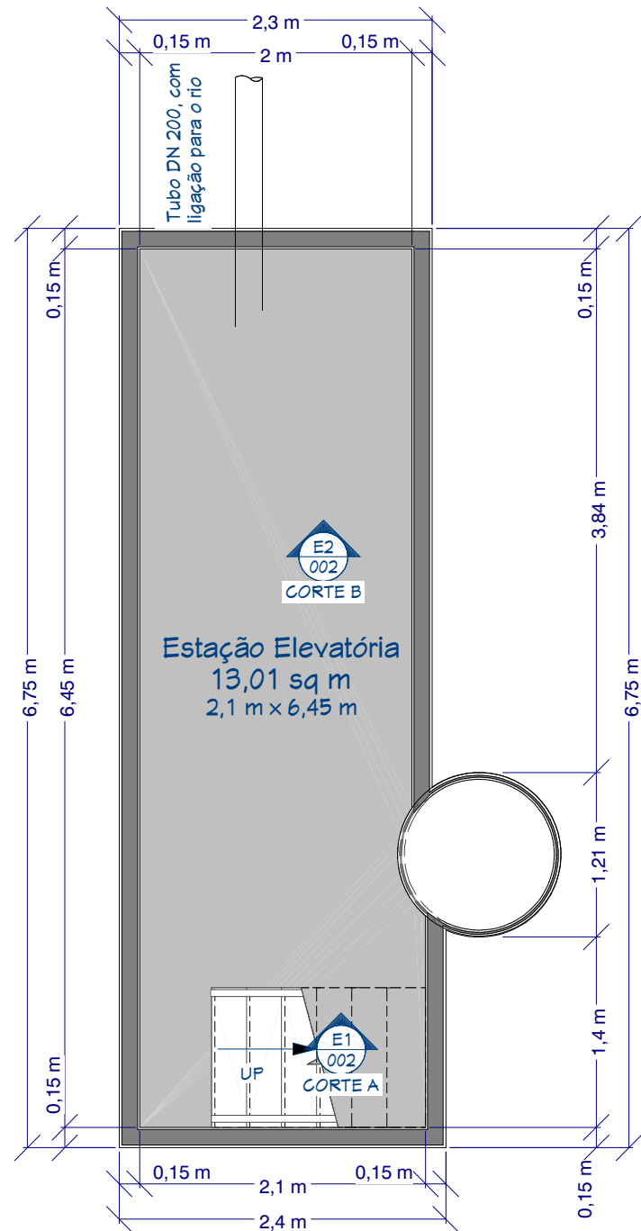
1 Planta Baixa - Subsolo 1 cm = 50 cm
