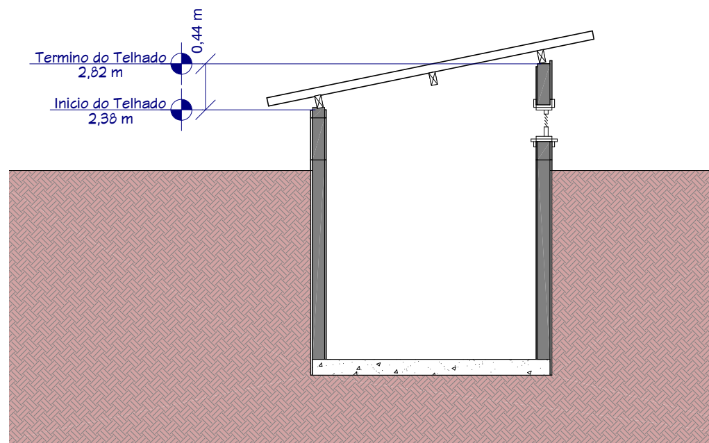
E2 CORTE B 1 cm = 50 cm
