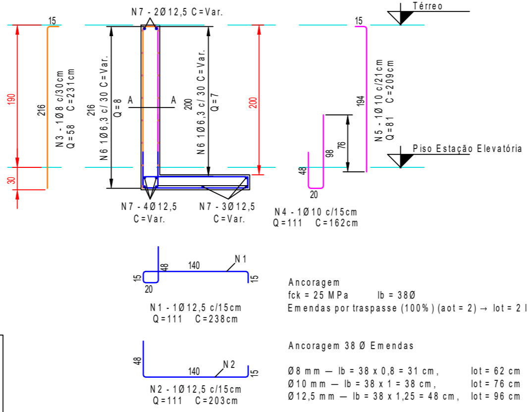
MURO DE FLEXÃO (M1 - M2 - M3 - M4 - M5)
