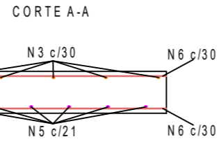
MURO DE FLEXÃO (M1 - M2 - M3 - M4 - M5)
