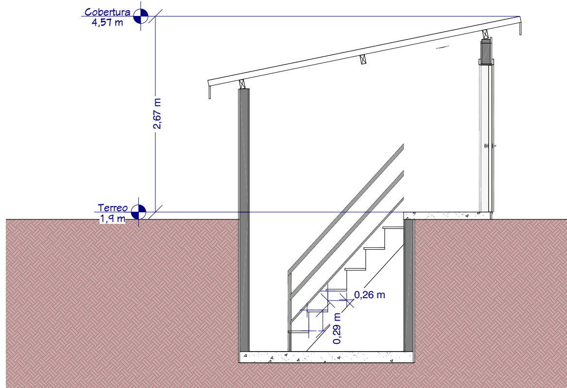
E1 CORTE A 1 cm = 50 cm
