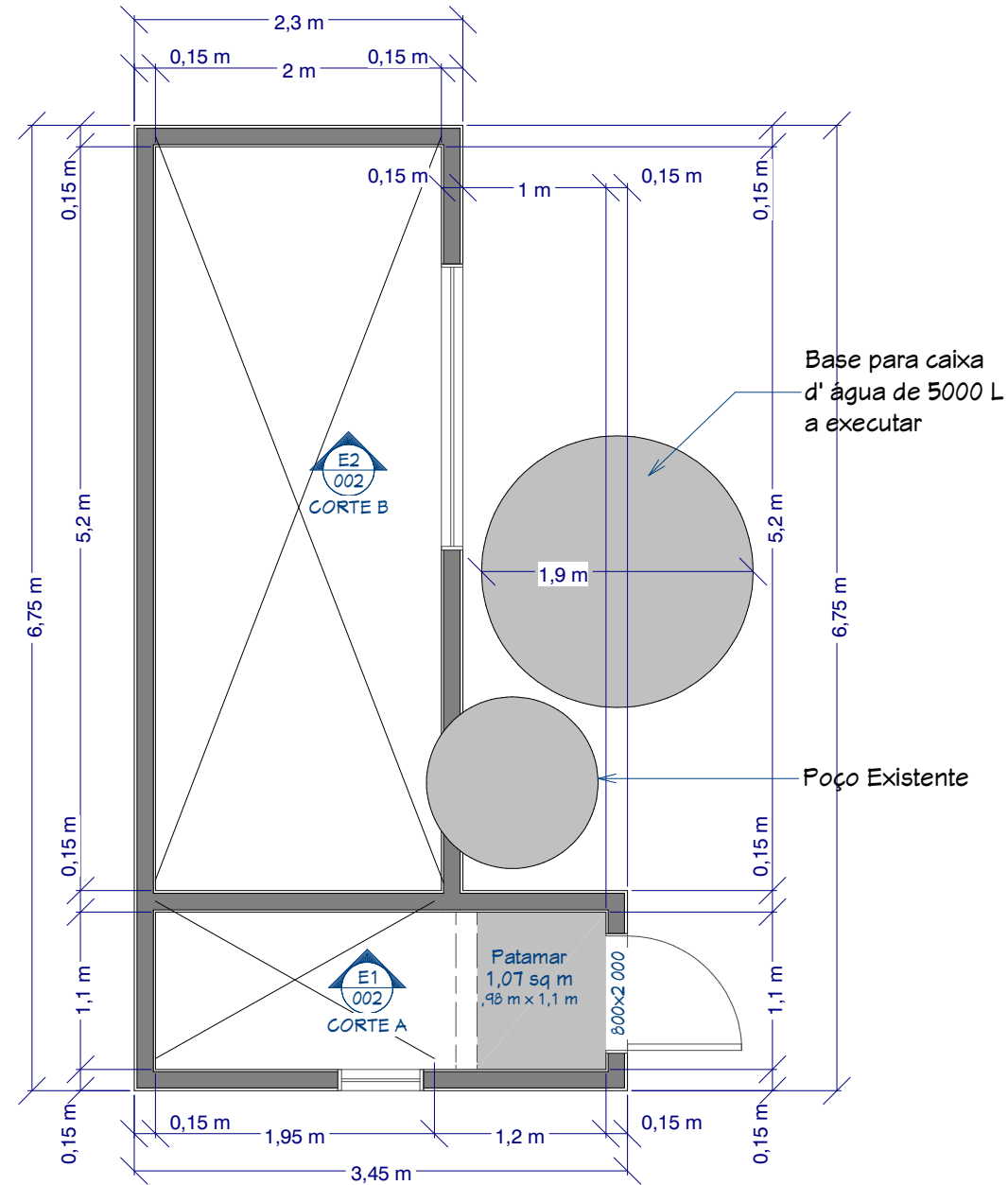
2 Planta Baixa - Térreo 1 cm = 50 cm
