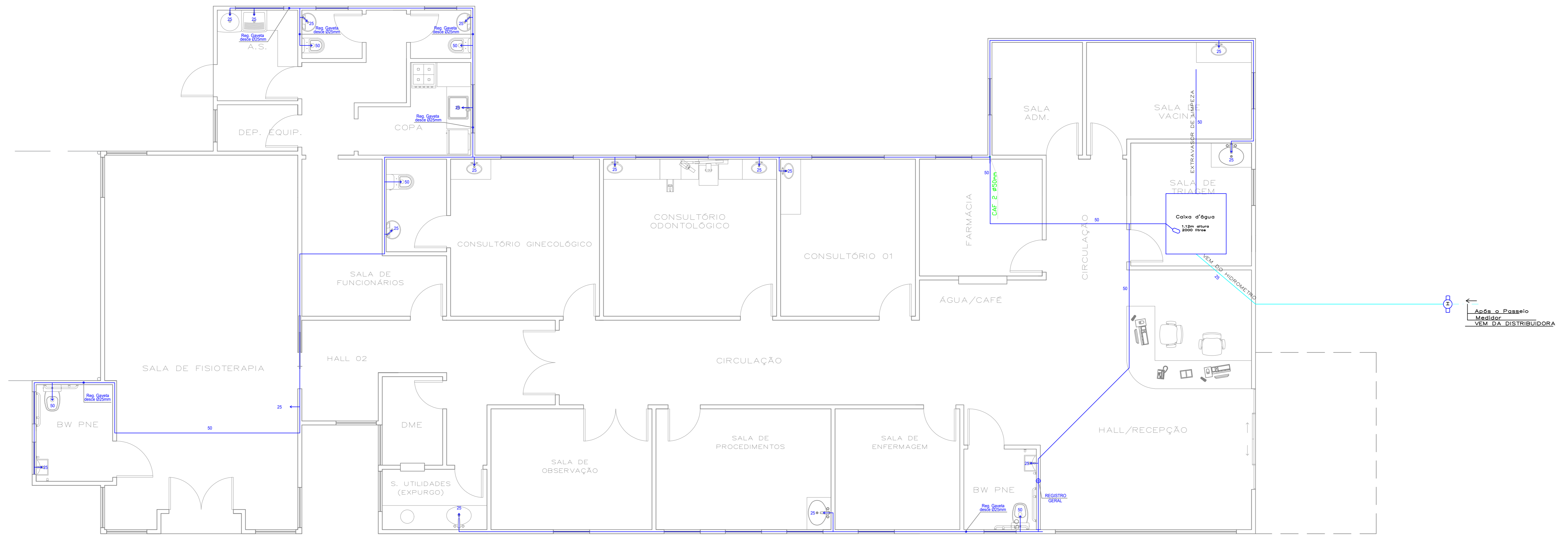
11 HIDRÁULICO ESCALA 1/50
