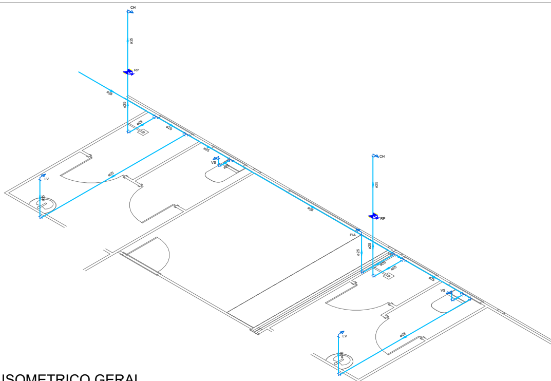
ISOMETRICO GERAL
