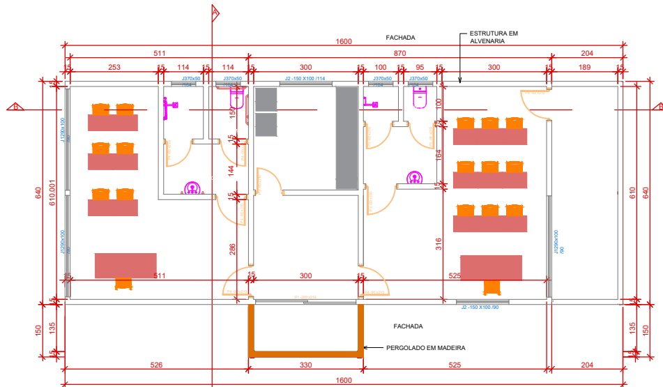
PLANTA BAIXA ÁREA TOTAL: 106,70M²
