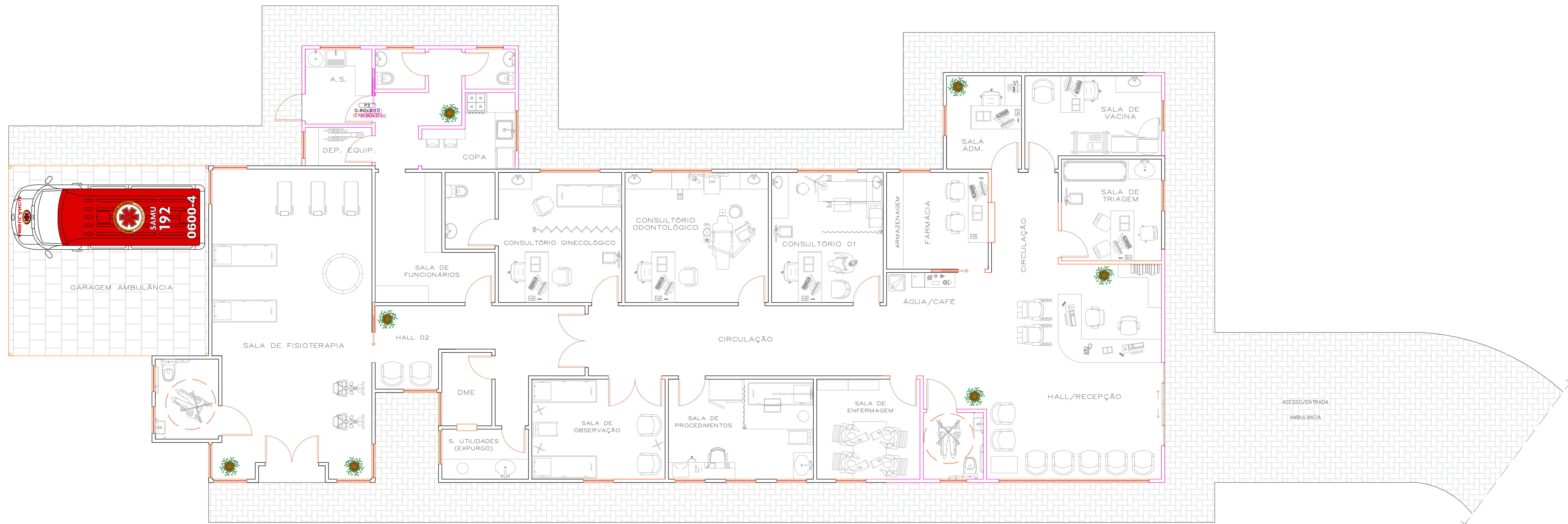
3 PLANTA DE LAYOUT ESCALA 1/50
