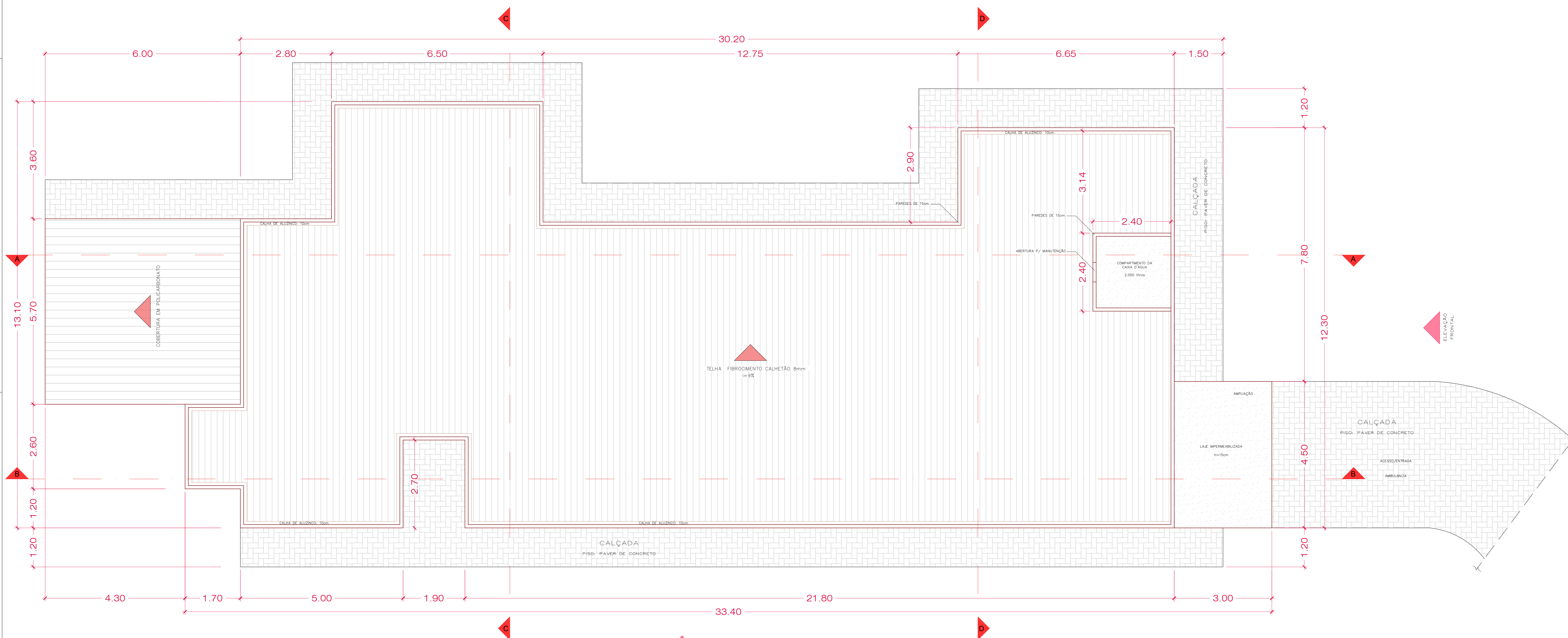
4 PLANTA DE COBERTURA ESCALA 1/50
