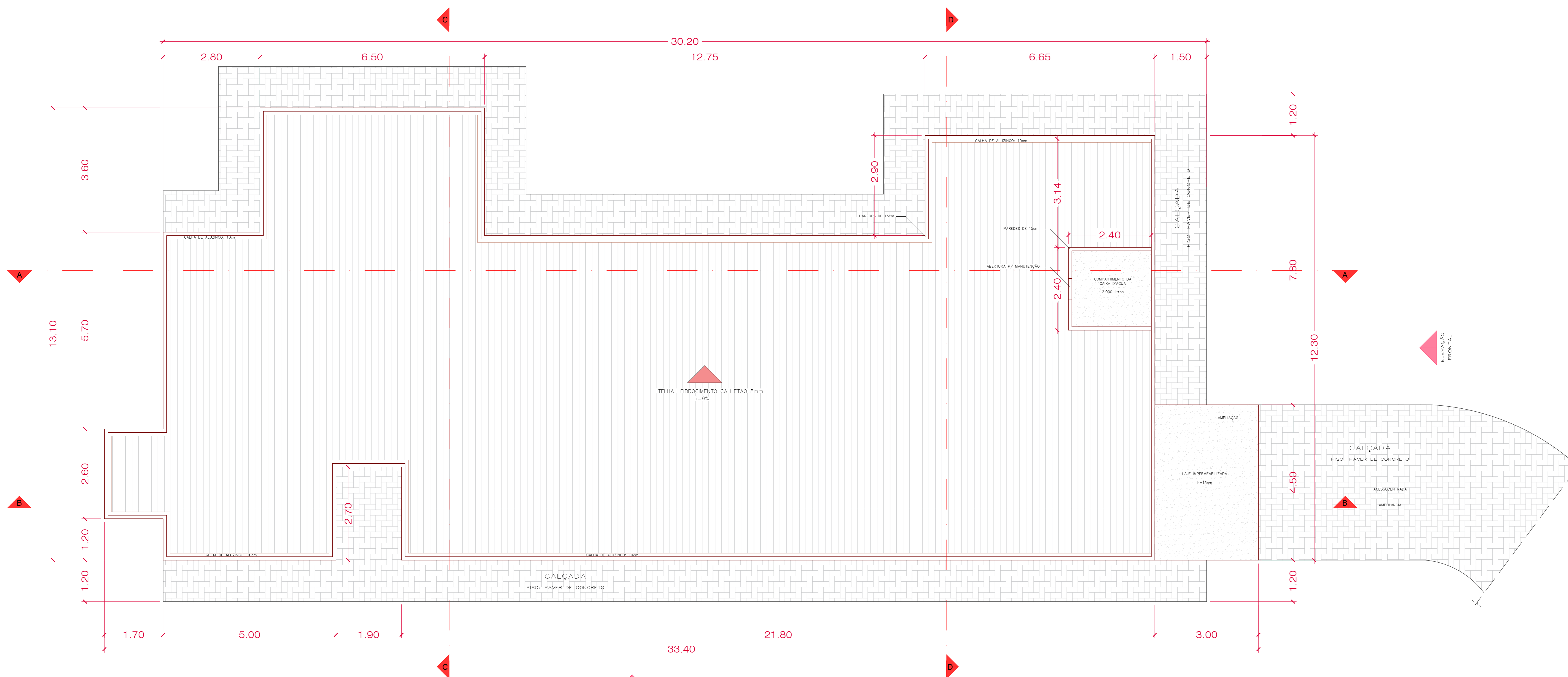
4 PLANTA DE COBERTURA ESCALA 1/50
