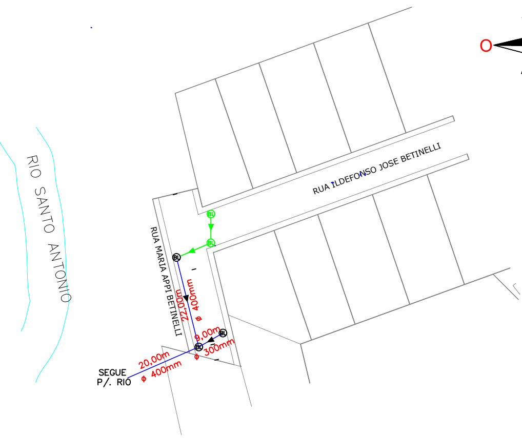
DRENAGEM ESC HOR. 1/1000
