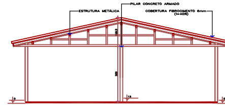
CORTE B B' ESC: 1/75
