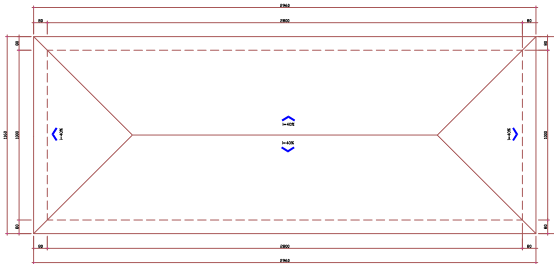
PLANTA COBERTURA ESC= 1/75
