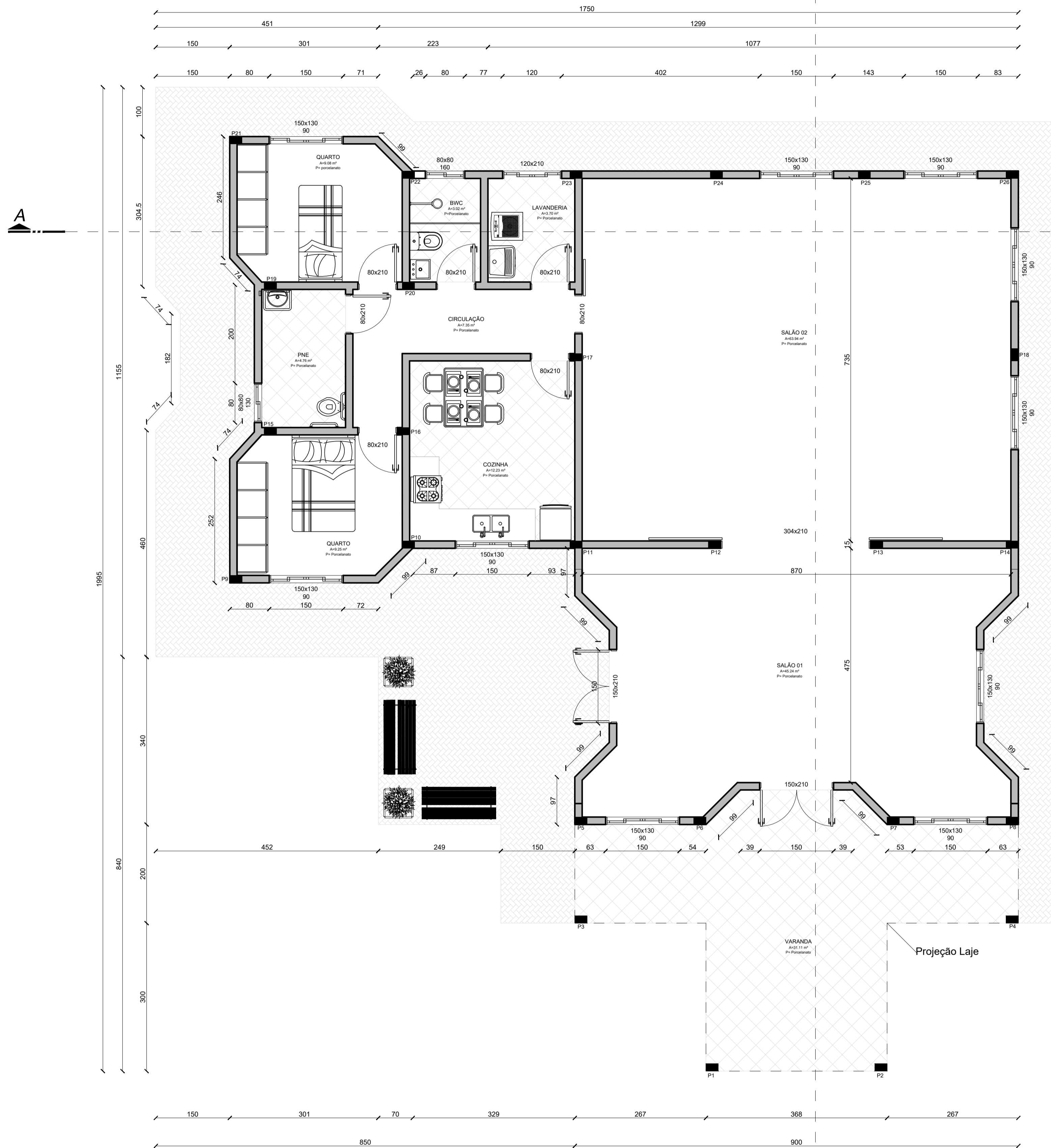
PLANTA BAIXA Escala 1/50 Área Total: 200.61 m 2
