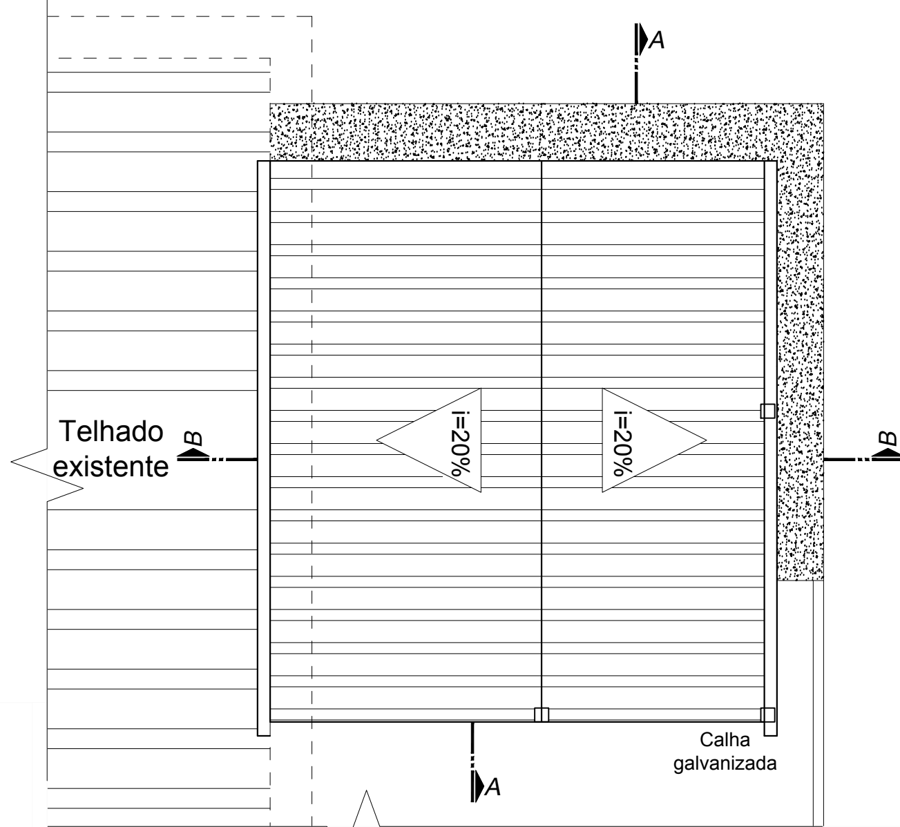
TELHADO esc.: 1/75
