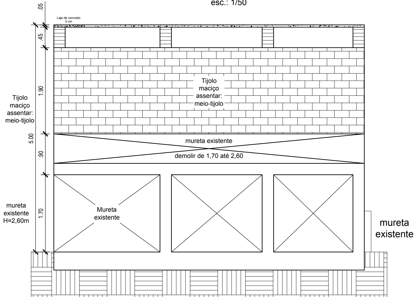
FACHADA LATERAL esc.: 1/50
