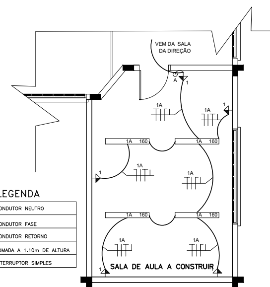
PLANTA BAIXA ELÉTRICO escala: 1 / 50 A=21,28 M2
